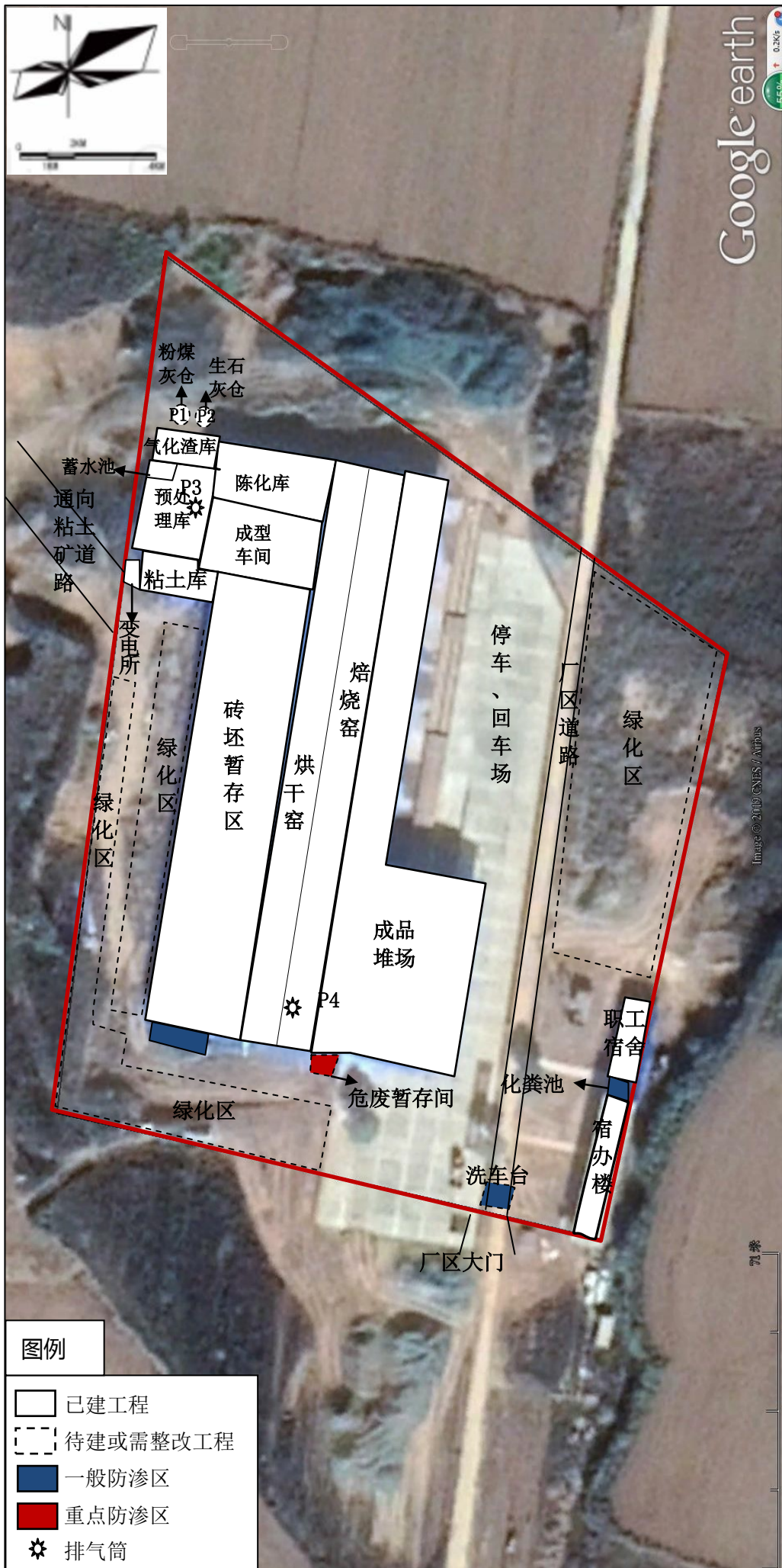
附图3 生产区平面布置及分区防渗示意图
