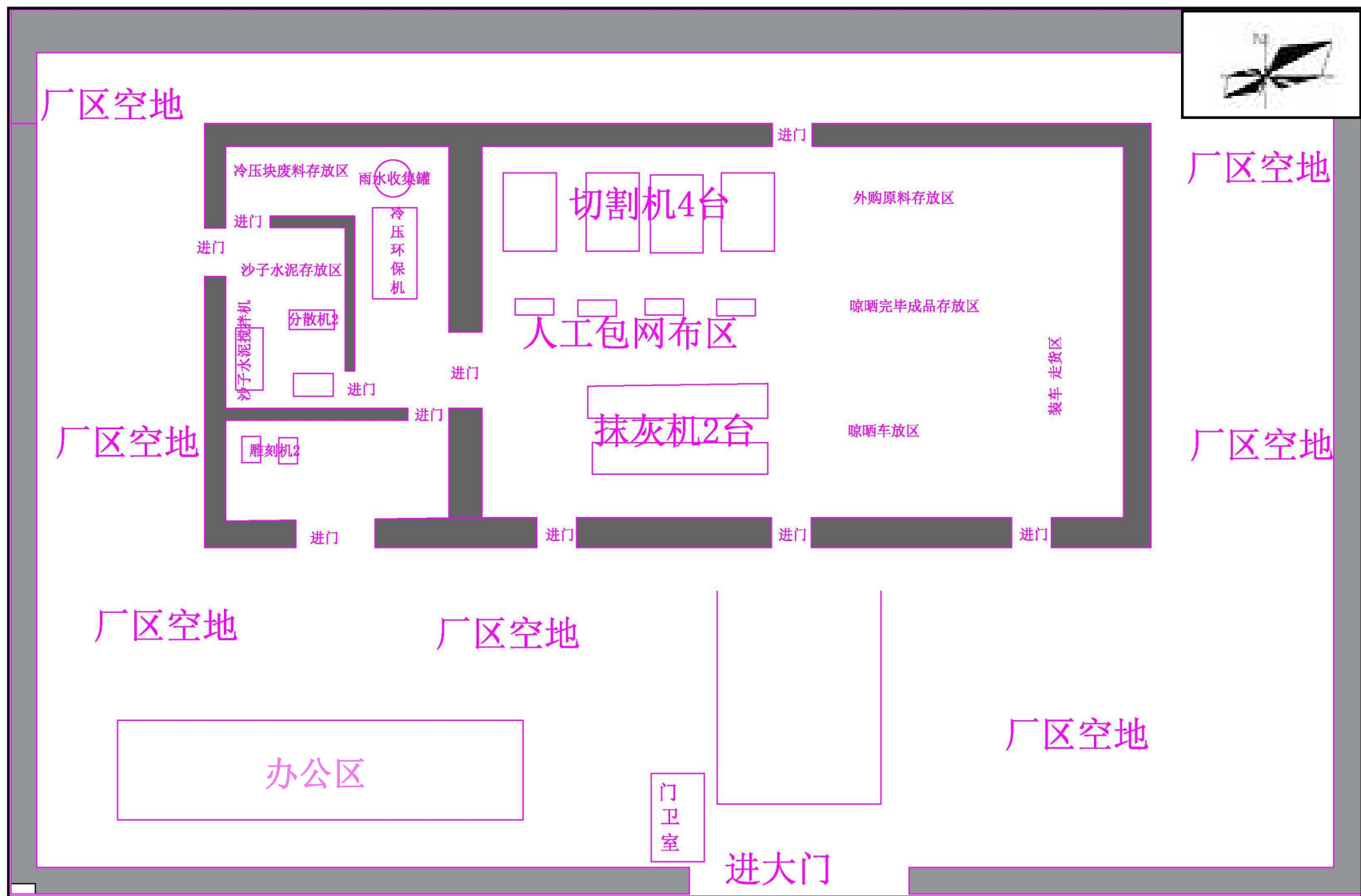
附图 4 平面布置图
