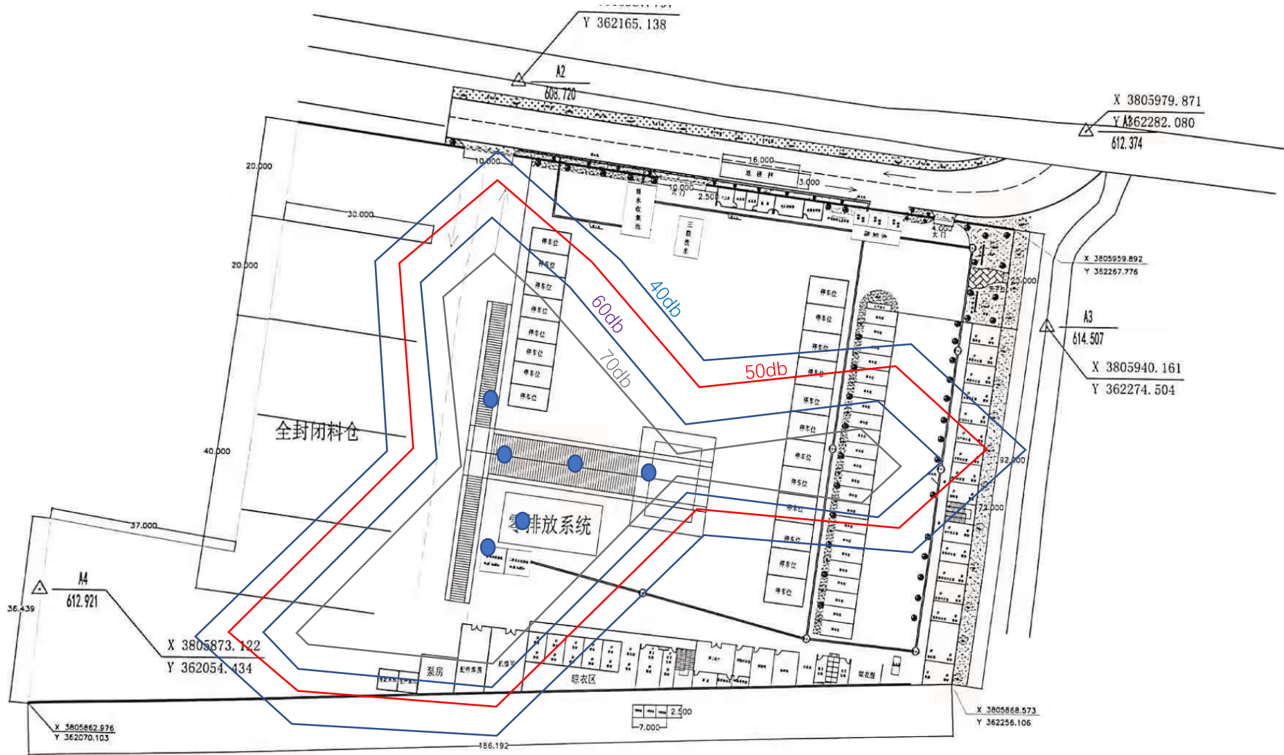
附图 5 噪声等值线图
