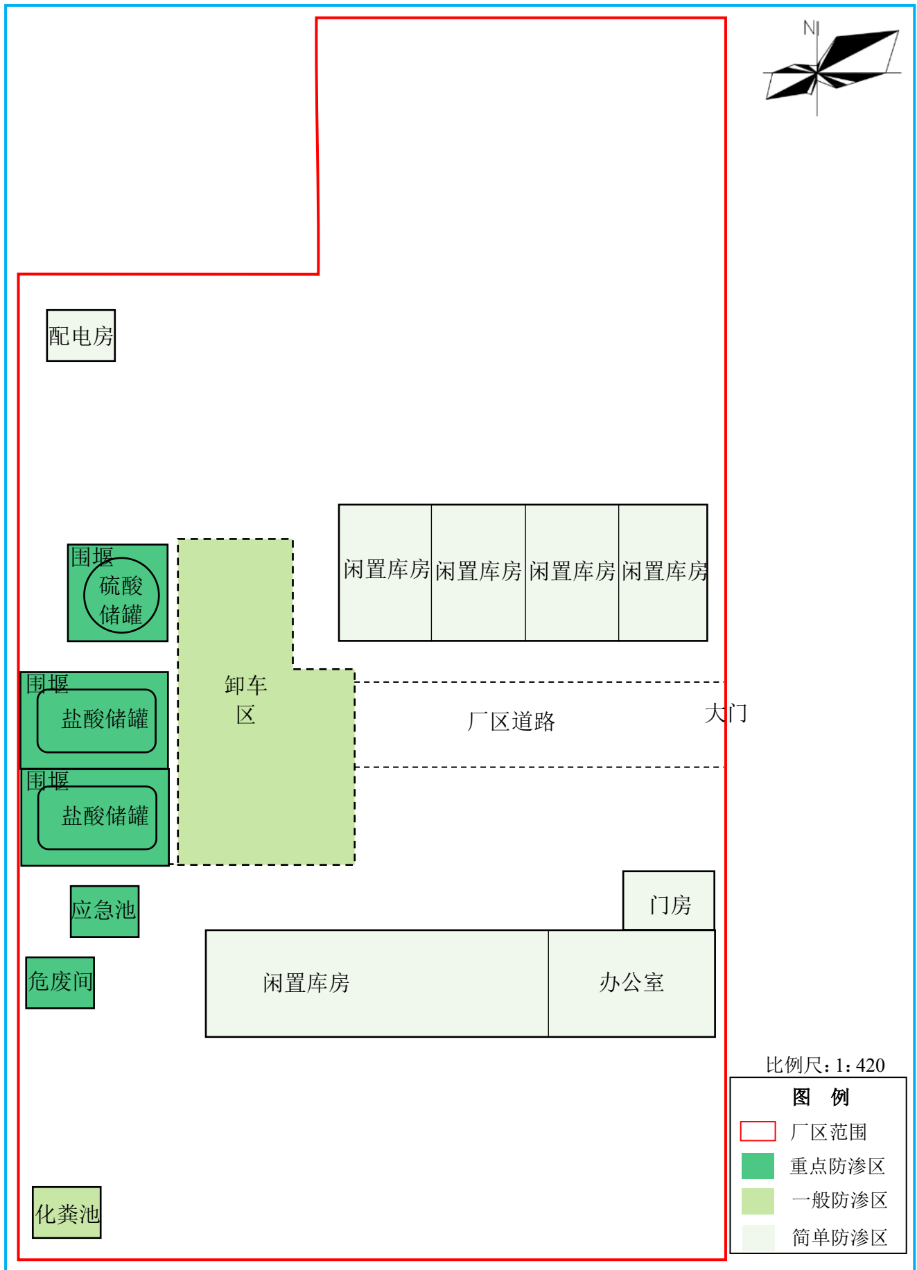
附图3 厂区分区防渗图
