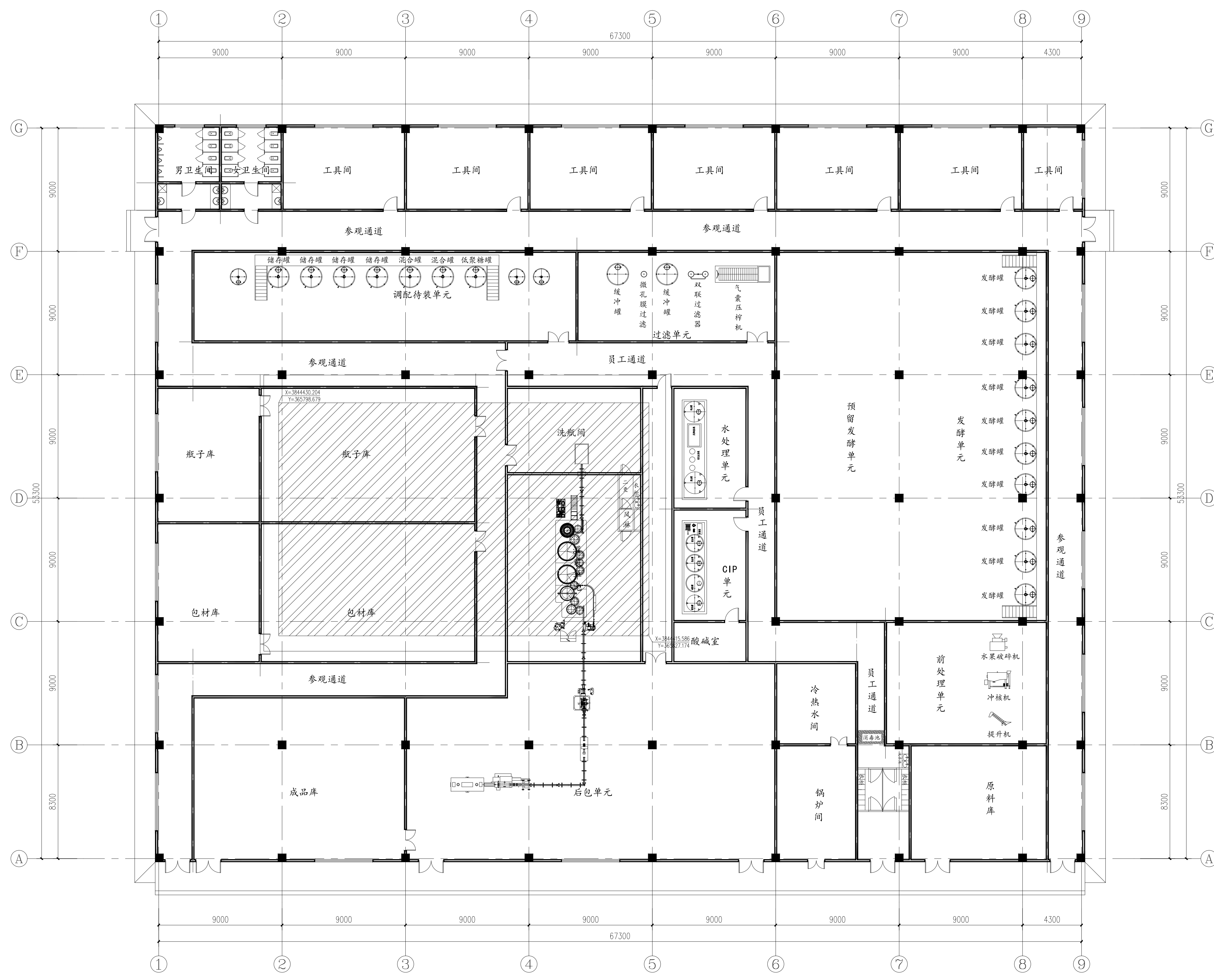
农产品深加工项目平面图 1:150
