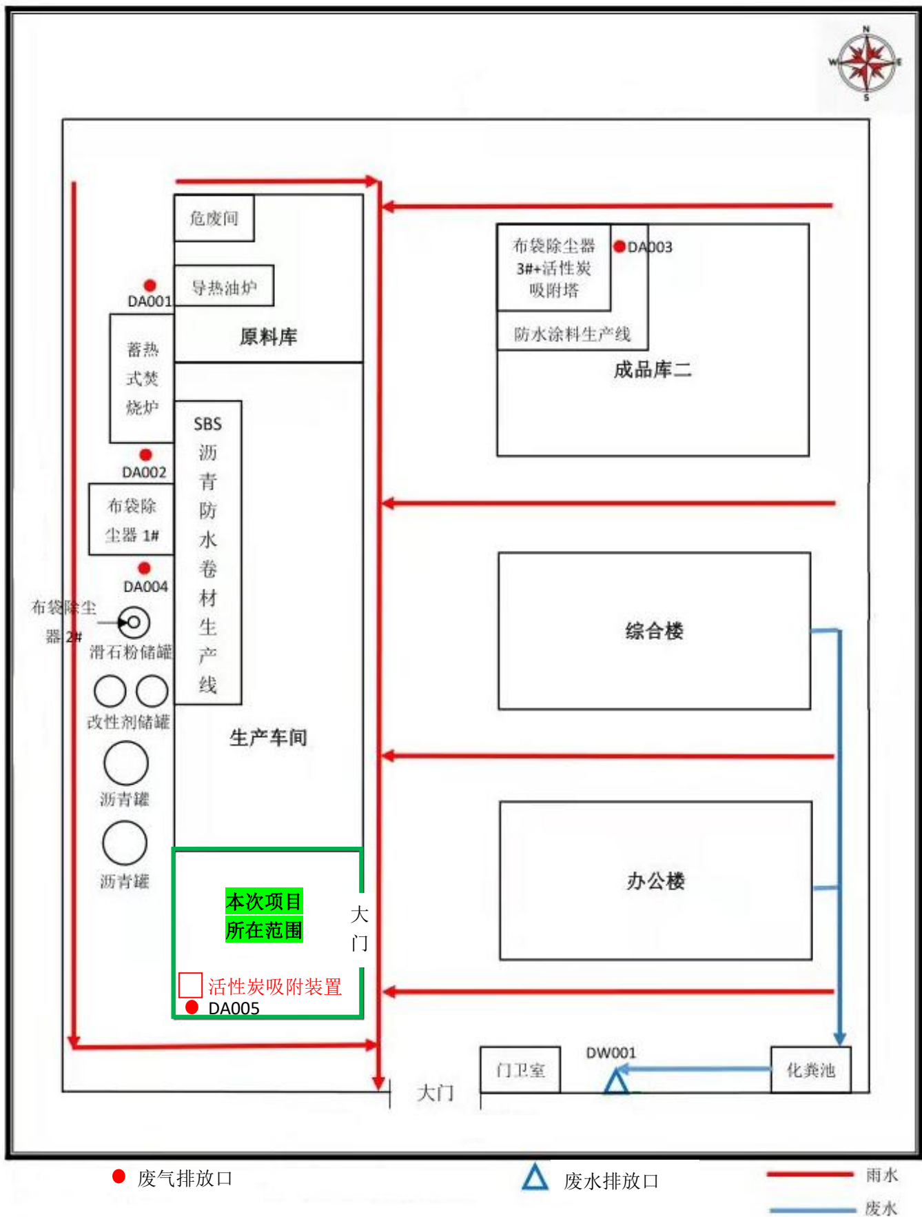
附图 3 总厂区平面布置图
