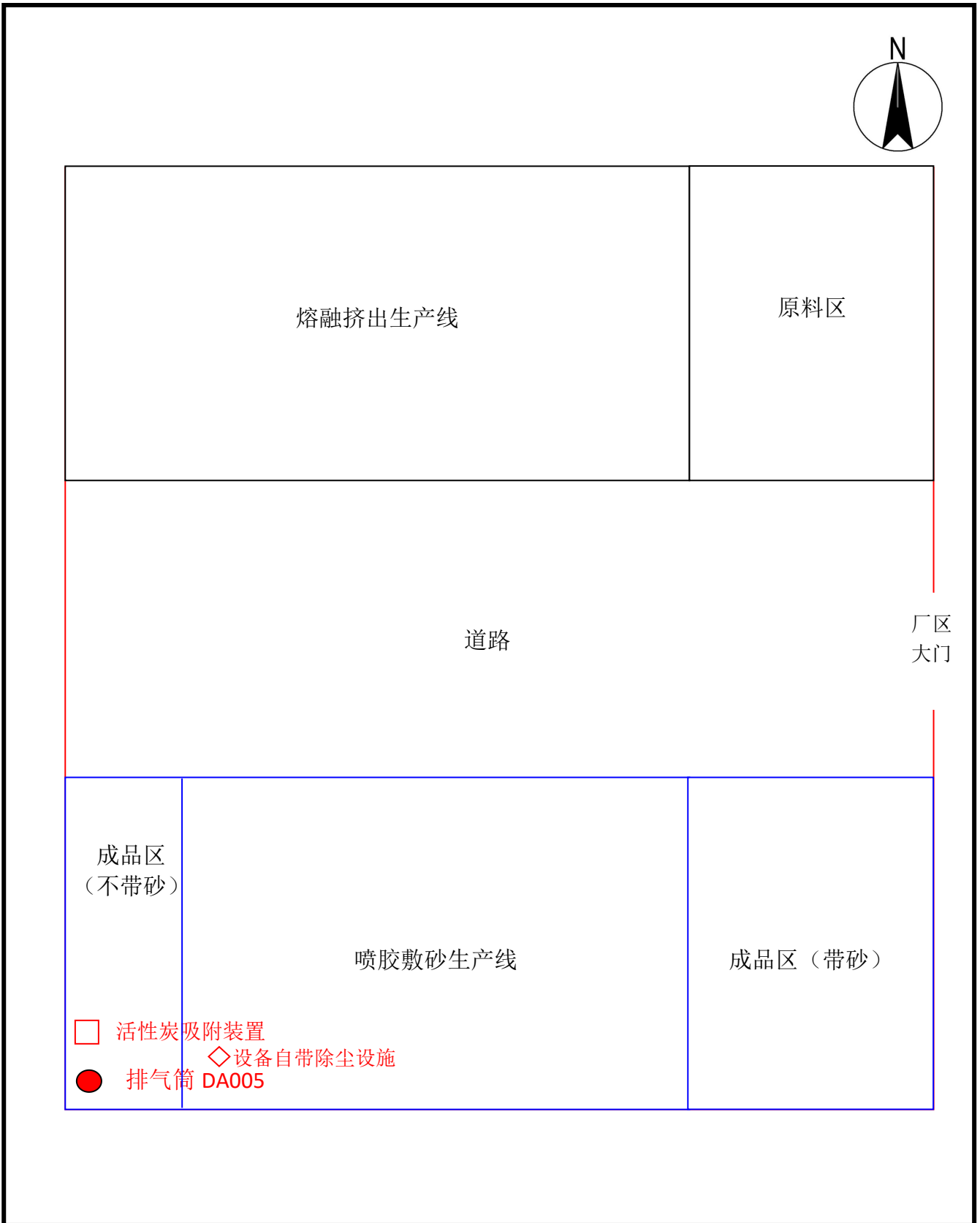
附图 4 本次项目平面布置图
