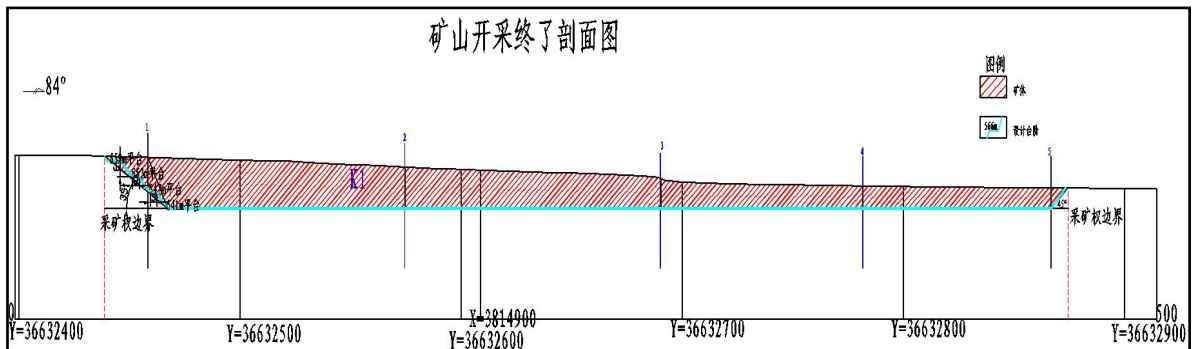
图 1.3-2 开采终了剖面图
