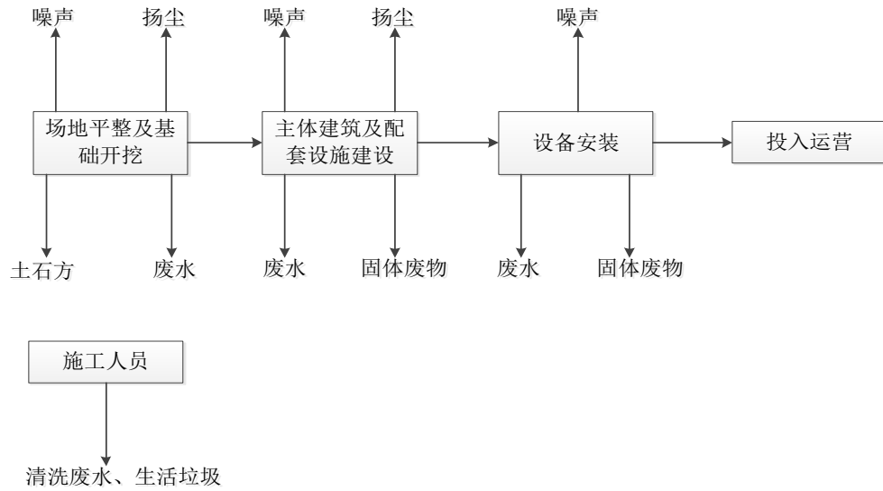
图 2-1 施工期工艺流程及产污环节图
