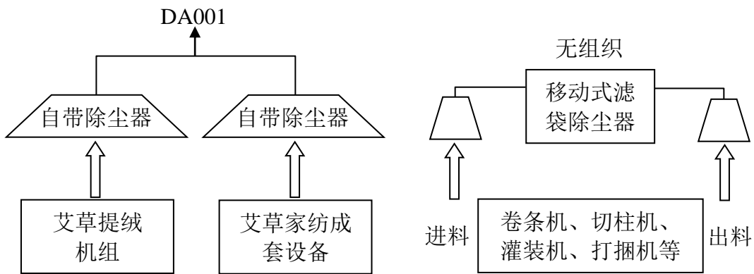
图 4-2 废气处理工序示意图
