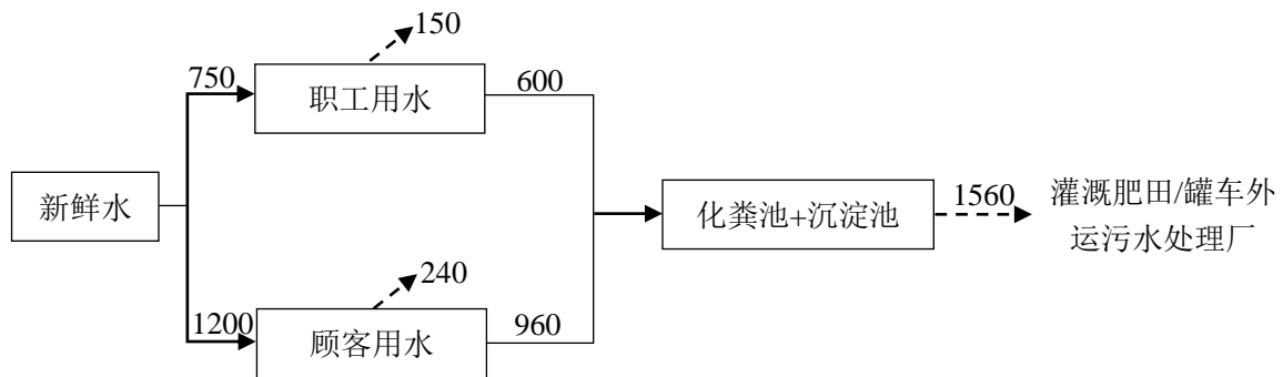
图 4-1 运营期用水量平衡图 单位：m 3 /a
