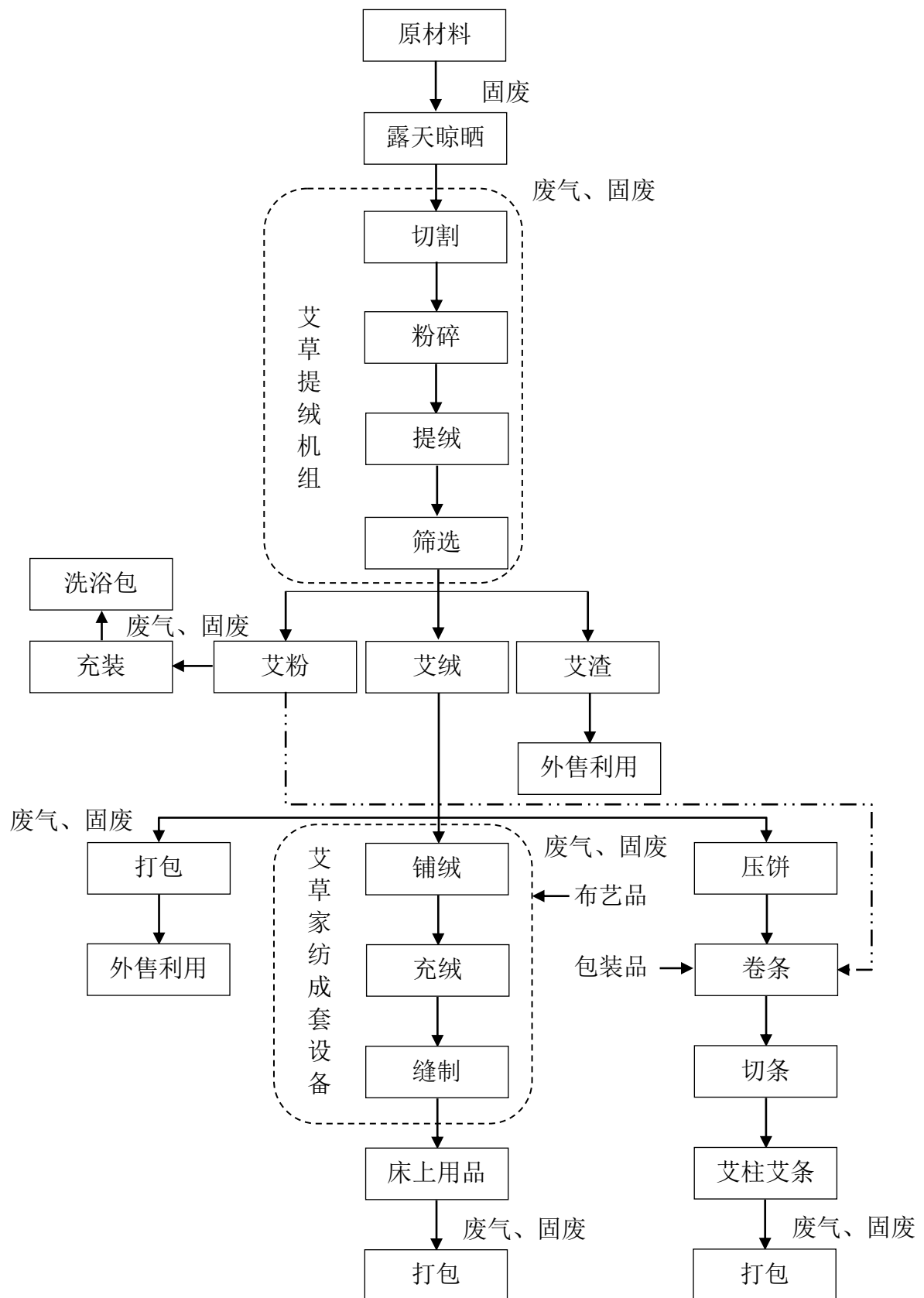
图 2-2 艾草制品生产工艺及产污环节图
